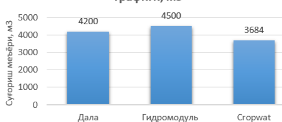
3-расм. Мавсум давомида фермернинг ўзи қўллаган одатий суғориш амалиёти, гидромодуль райони тавсияси ва модель ишлаб чиққан суғориш меъёрларининг таққослаш графиги
