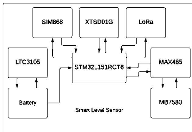
8-расм. Ақлли сатҳ сенсорнинг тузилиши
