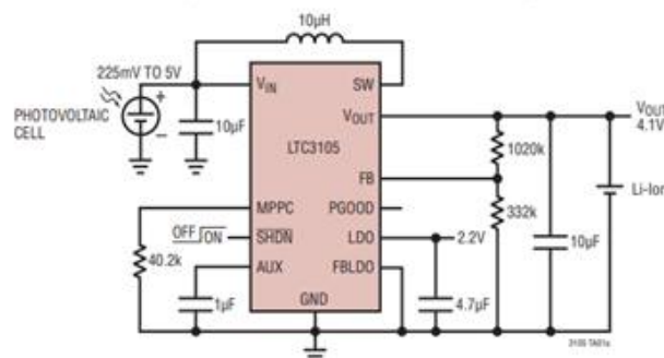
3-расм. Батареякани зарядлаш учун LTC3105 конвертерининг уланиш схемаси
