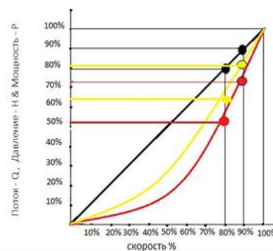
Рис 5. График изменения основных параметров центробежного насоса при уменьшении скорости на 10% ( f=45\text{Гц} ) и на 20% ( f=40\text{Гц} ).
