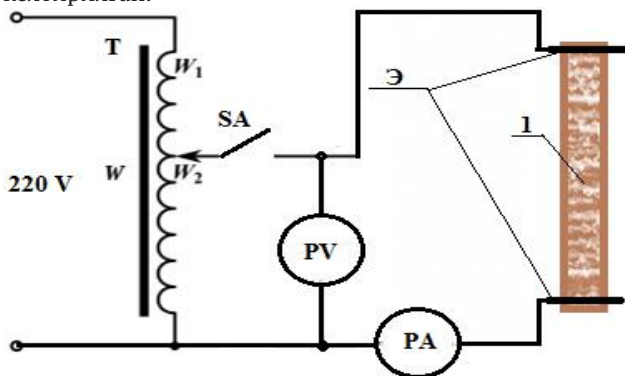
1 – узум қаламчаси; Э – электродлар; РА – миллиамперметр; PV – вольтметр
